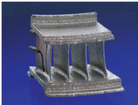
Leitschauflersegment mit integrierten Messkanälen (mit freundlicher Genehmigung von MTU)
